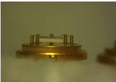
Bauelement montiert: Mikro-Gassensor
