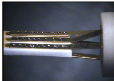
Widerstandsschweißung einer Sensor-Zelle
