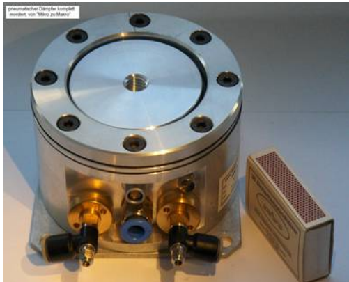
Abb. 3: pneumatisches Dämpfungssystem
