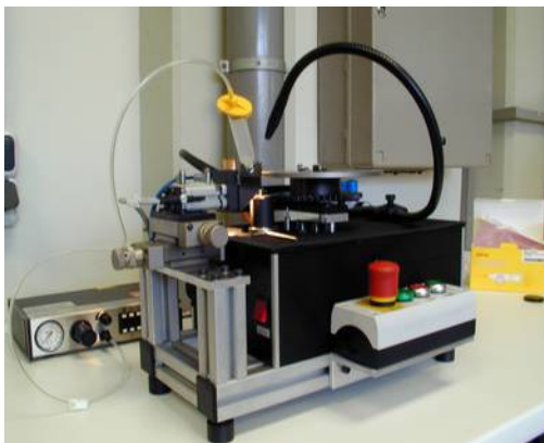
Abb. 5: Lackiergerät für optische Linsen
